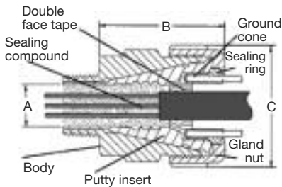
With conduit
